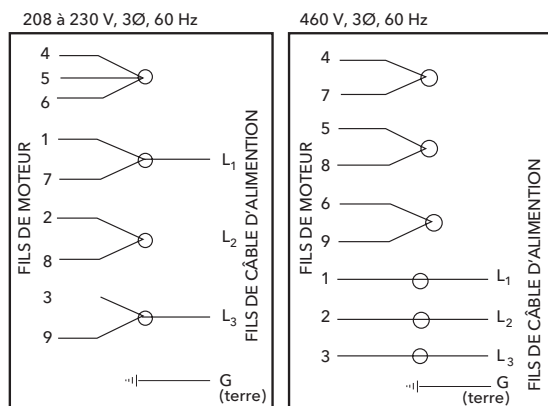
SCHÉMAS DE CÂBLAGE DES MOTEURS TRIPHASÉS
